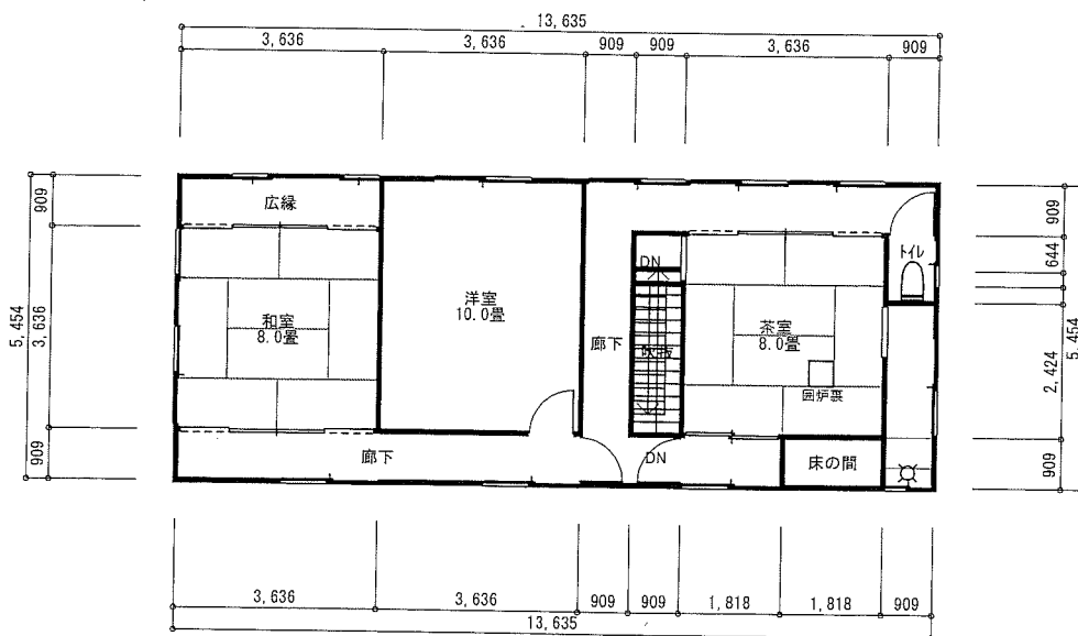
2階 縮尺 1/150
